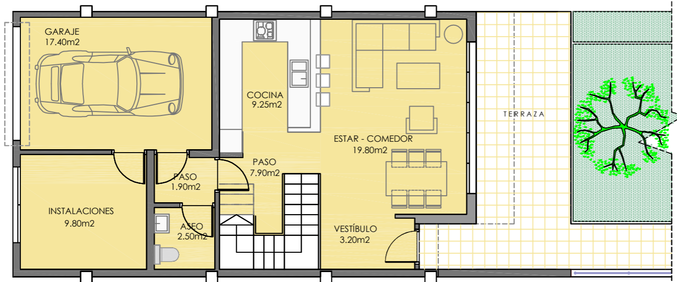
SÓTANO - BAJA
